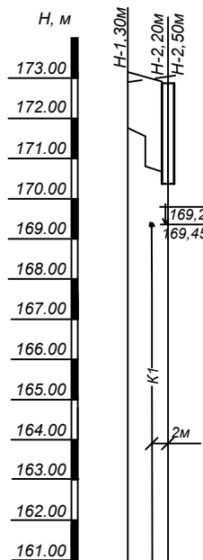
Профиль -В1-, (водопроводный ввод в ж/д №2) Мг 1:500, Мв 1:100
