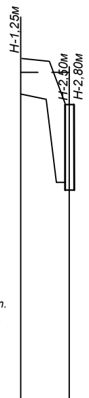
Профиль -В1-, (водопроводный ввод в ж/д №6) Мг 1:500, Мв 1:100
