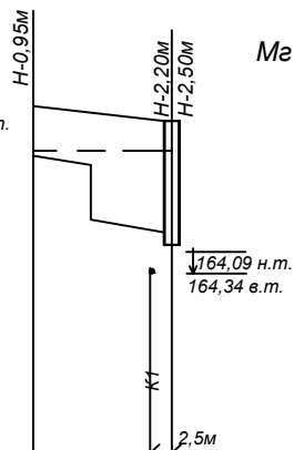
Профиль -В1-, (водопроводный ввод в ж/д №4) Мг 1:500, Мв 1:100
