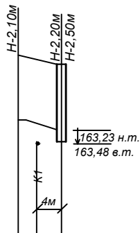
Профиль -В1-, (водопроводный ввод в ж/д №7) Мг 1:500, Мв 1:100
