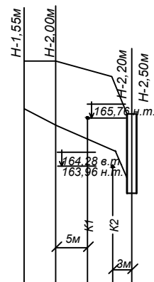
Профиль -В1-, (водопроводный ввод в ж/д №6) Мг 1:500, Мв 1:100
